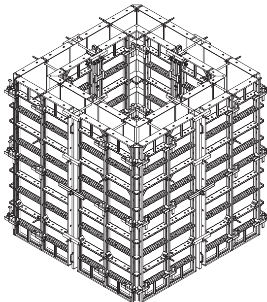
Rys. 7.6 – Przykład zmontowanego szalunku szyby windowego
