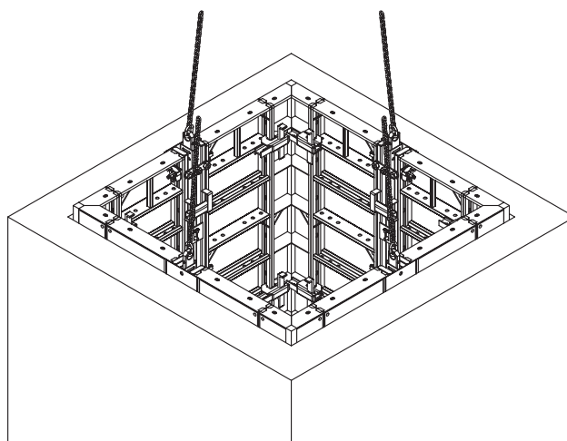
Rys. 7.12 – Demontaż segmentu wewnętrznego
