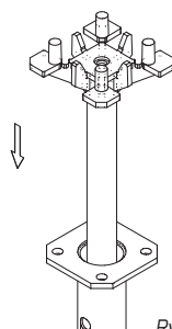
Rys. 14.8 – Podparcie głowicą wsporczą z nakładką głowicy w wnożu ściany
