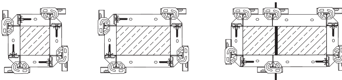
Formowanie słupów - płyty MIDI BOX i zamki szalunkowe
