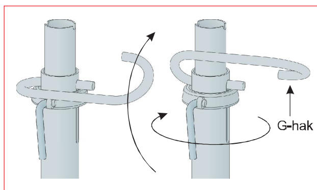
Kolejność postępowania przy odciażaniu podpory przy użyciu G-haka
