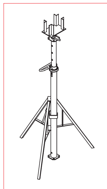
Schemat montażu podpory w trójnóg
