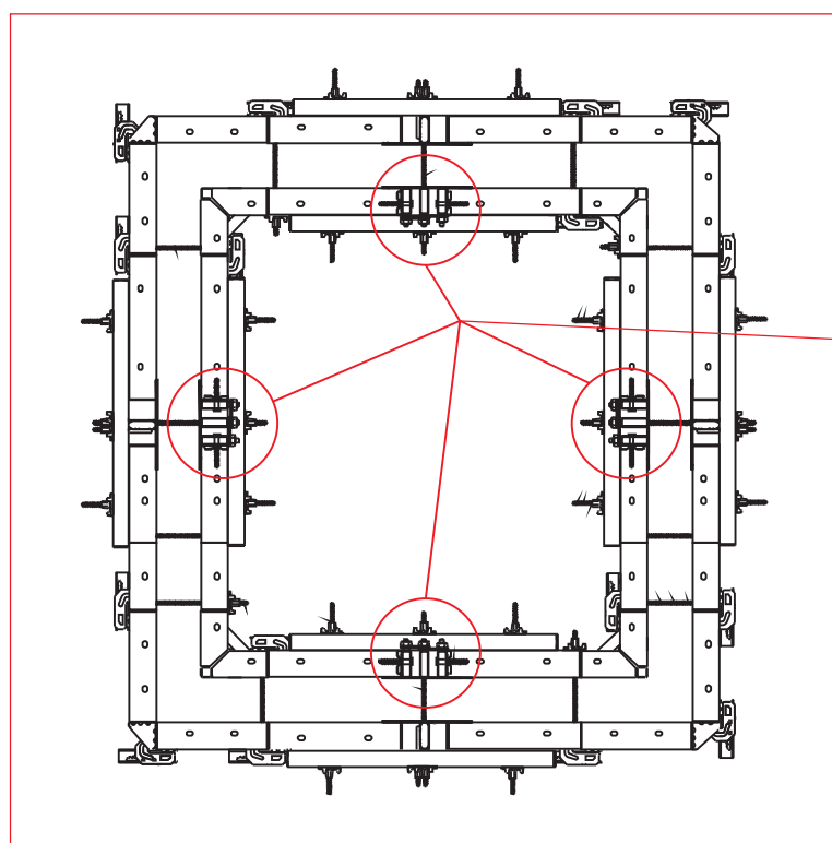
Szalunek szybu windowego - schemat
