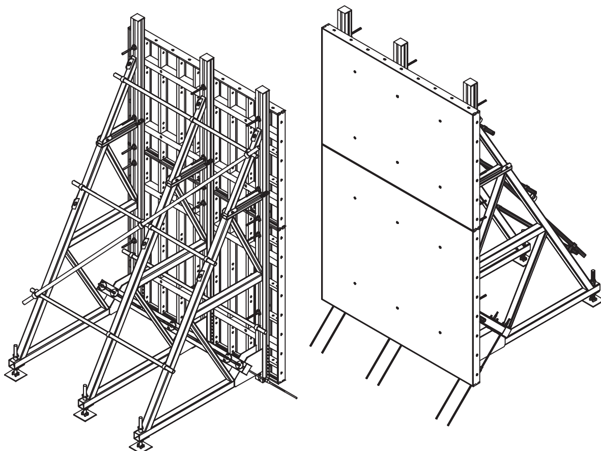
Schemat szalunku jednostronnego z wykorzystaniem kozłów podporowych typu A i B
