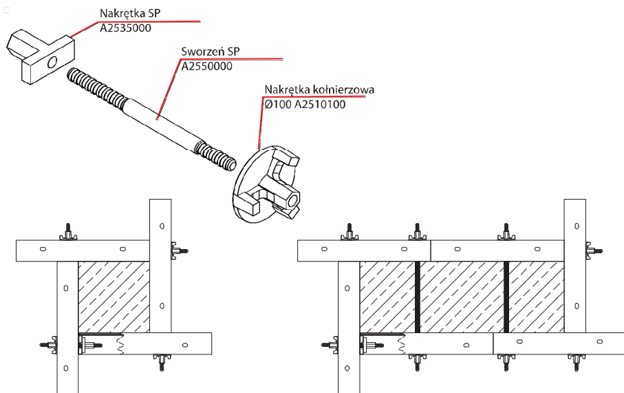
Schemat łączenia płyt
