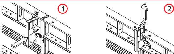
Zawiesie transportowe - zastosowanie
