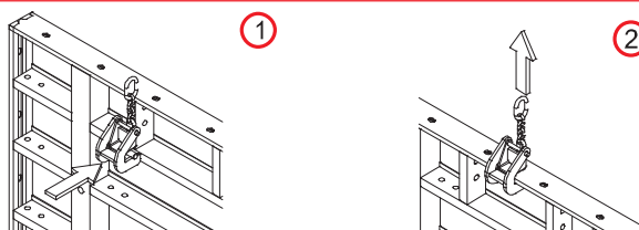
Zawiesie transportowe - przykład montażu
