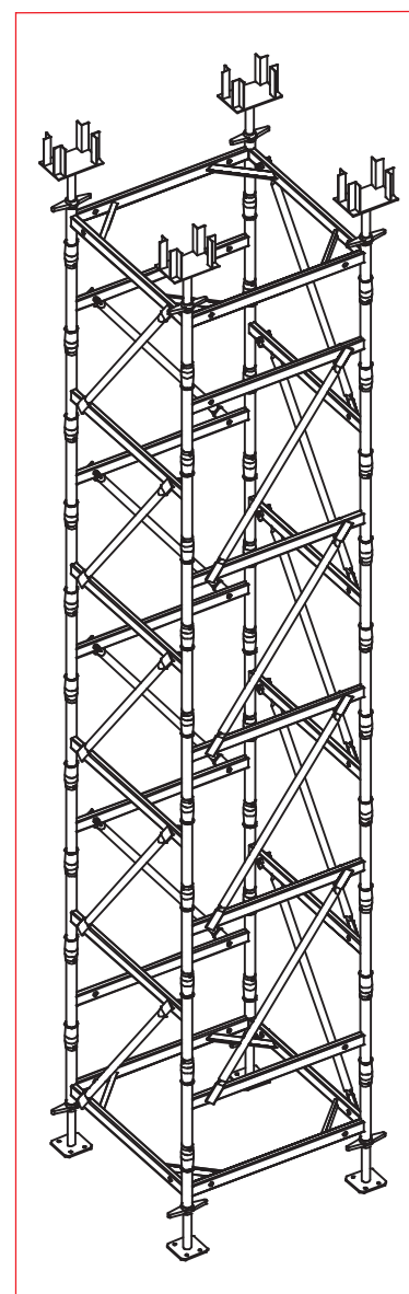
Wieża podporowa S10 - schemat
