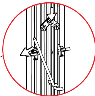
Odblokowanie szalunku szybu windowego
