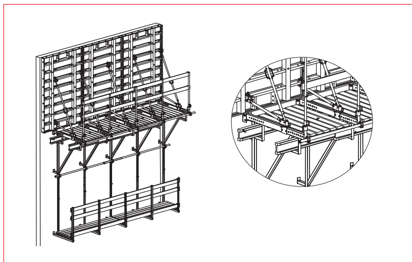
Schemat - szalunek wspinający
