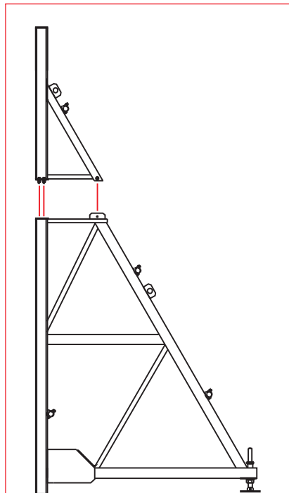
Kozły podporowe typu A i B - schemat montażu
