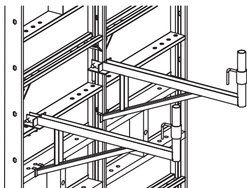
Schemat - montaż pomostów roboczych
