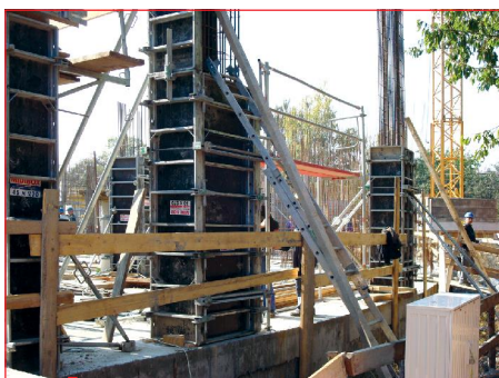
Formowanie słupów - płyty MIDI BOX i zamki szalunkowe
