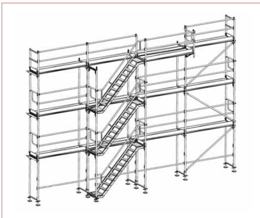
▪ Widok całości - klatka jednozabiegowa
