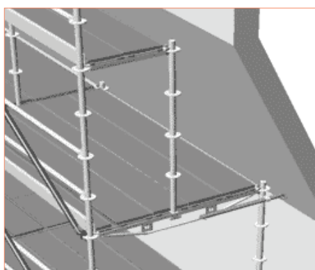
Rys. 3.48 – Zastosowanie łącznika dźwigara
