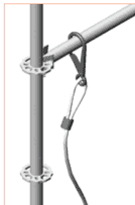
Rys. 3.9 – Mocowanie do rygli
