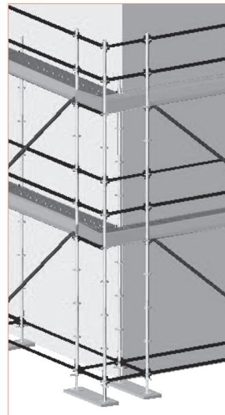
Rys. 3.26 – Narożnik wykonany za pomocą czterech stojaków
