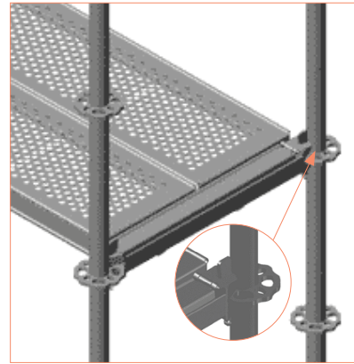
Rys. 3.21 – Etap 4 – Zaciśnąć
