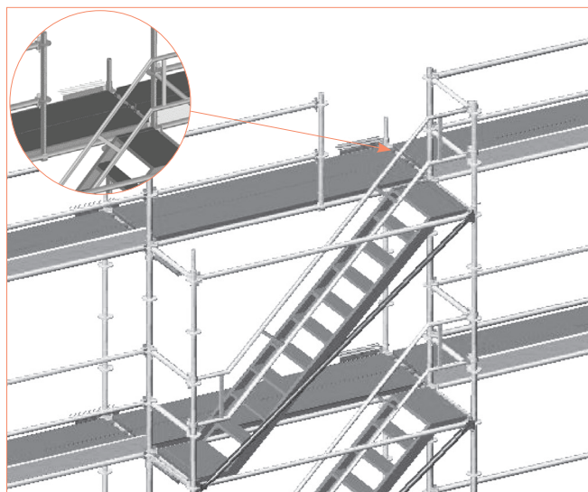
Rys. 3.78 – Wyjście z klatki przykład nr 2
