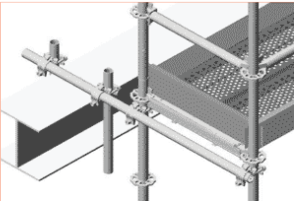
Rys. 3.33 – Kotwienie do belek poziomych
