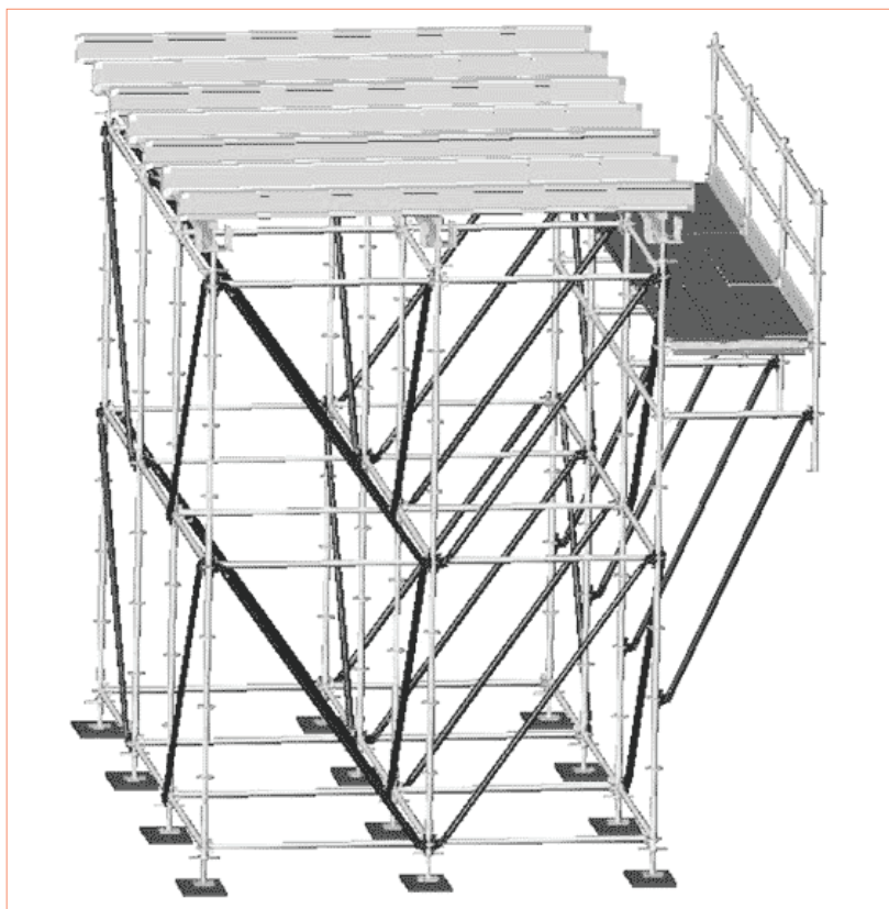
Rys. 3.65 – Rusztowanie ROTAX Plus w ustawieniu stropowym
