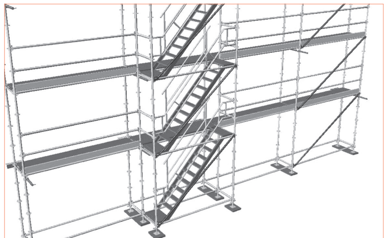
Rys. 3.76 – Zewnętrzna klatka schodowa jednozabiegowa
