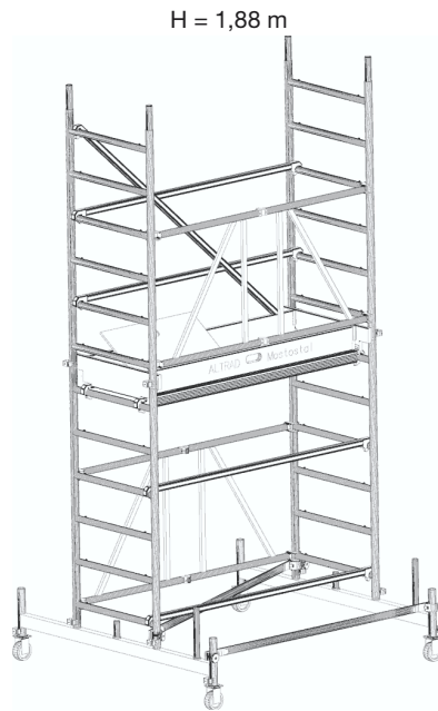
MP Mini 602
