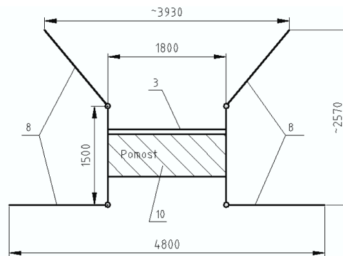
Ustawienie niesymetryczne
