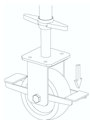
Koło odblokowane
