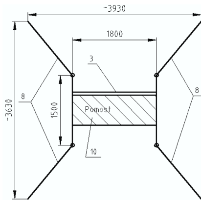
Ustawienie symetryczne
